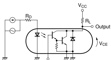
Fig.15 周波数特性の測定回路
