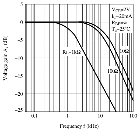
Fig.14 周波数特性
