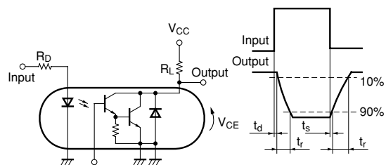
Fig.13 応答時間の測定回路
