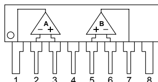
NJM2903L/2403L
