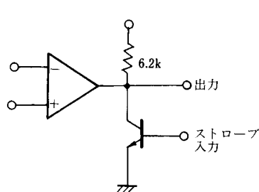
出力ストロープ回路
